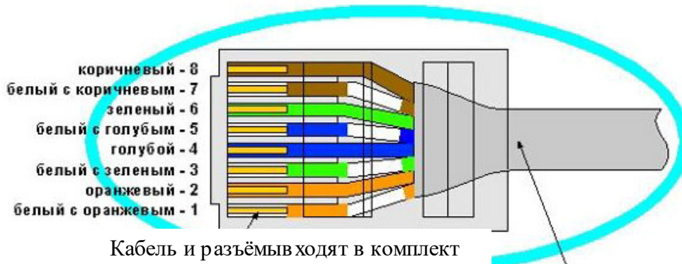
Вид сверху со стороны контактов
